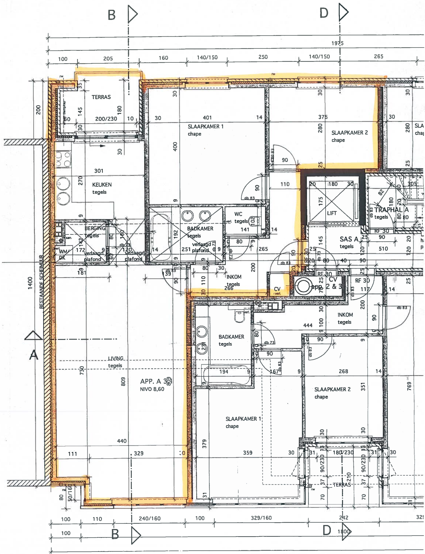
VERDIEPING 3 schaal 1/50
